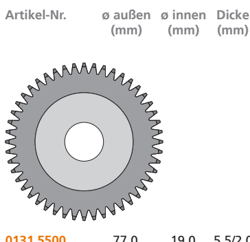
Artikel-Nr. 0131.5500 ø außen (mm) 77,0 ø innen (mm) 19,0 Dicke (mm) 5,5/2,0
