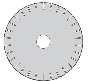
Artikel-Nr. 0139.0800 ø außen (mm) 110,0 ø innen (mm) 19,0 Dicke (mm) 0,80
