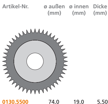
Artikel-Nr. 0130.5500 ø außen (mm) 74,0 ø innen (mm) 19,0 Dicke (mm) 5,50
